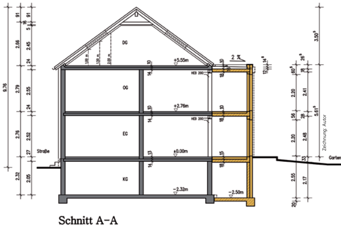
Abbildung 1: Systemschnitt der angestrebten zweieinhalbgeschossigen Erweiterung
